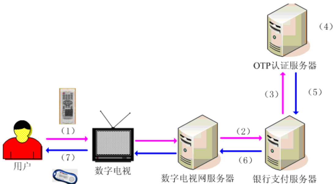
图3 认证过程
